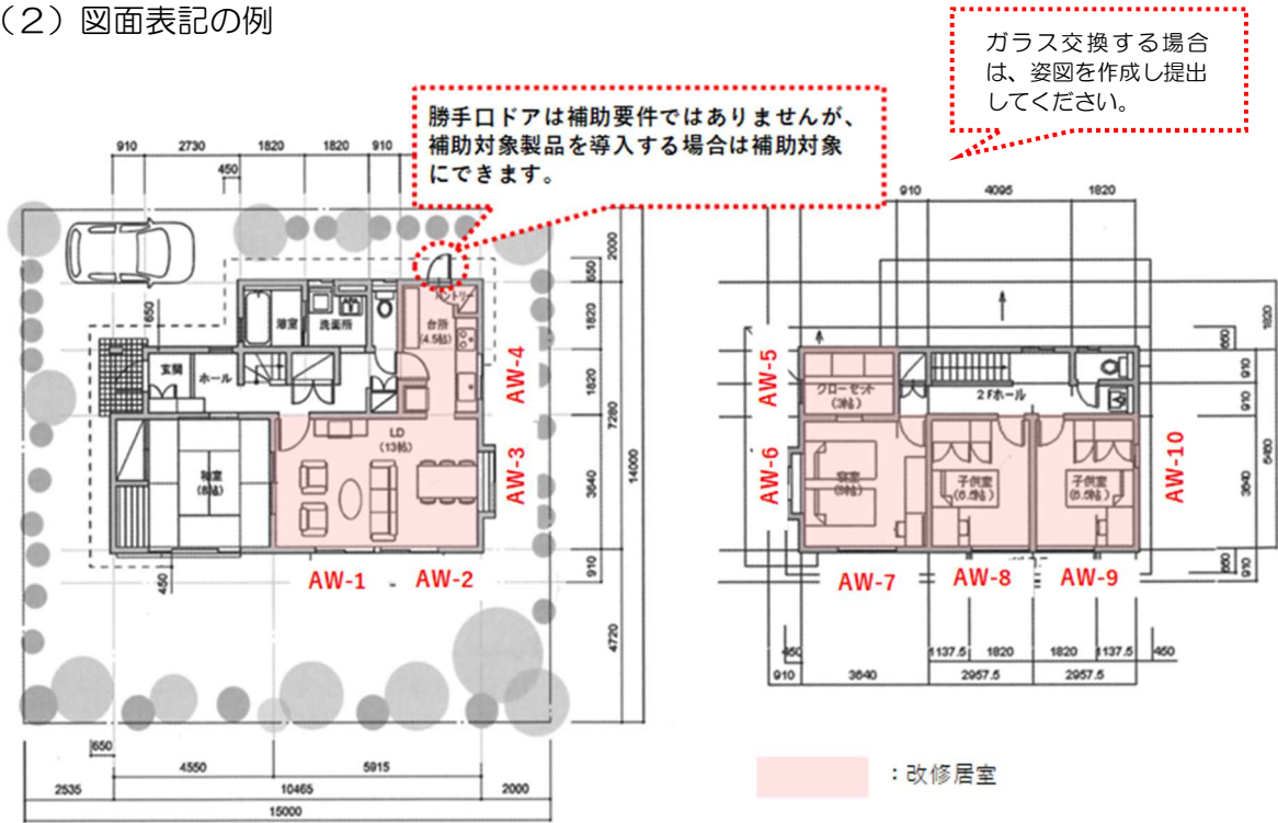
図9 窓改修寸法
